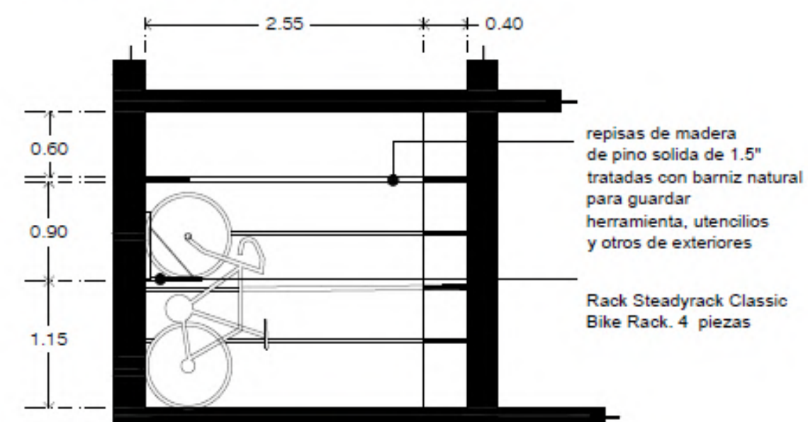
ALZADO INTERIOR B-B'
