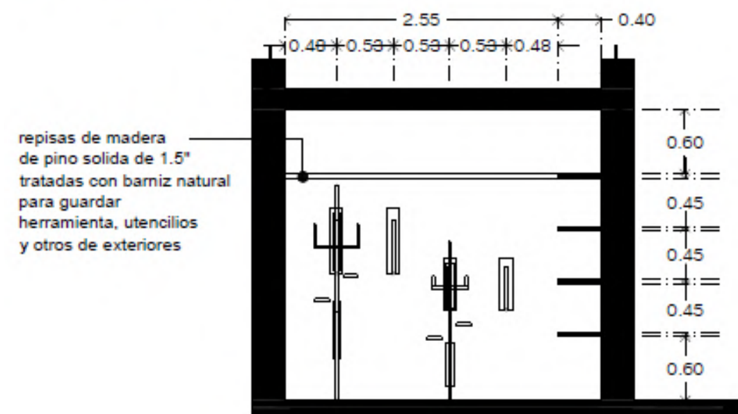
ALZADO INTERIOR A-A'
