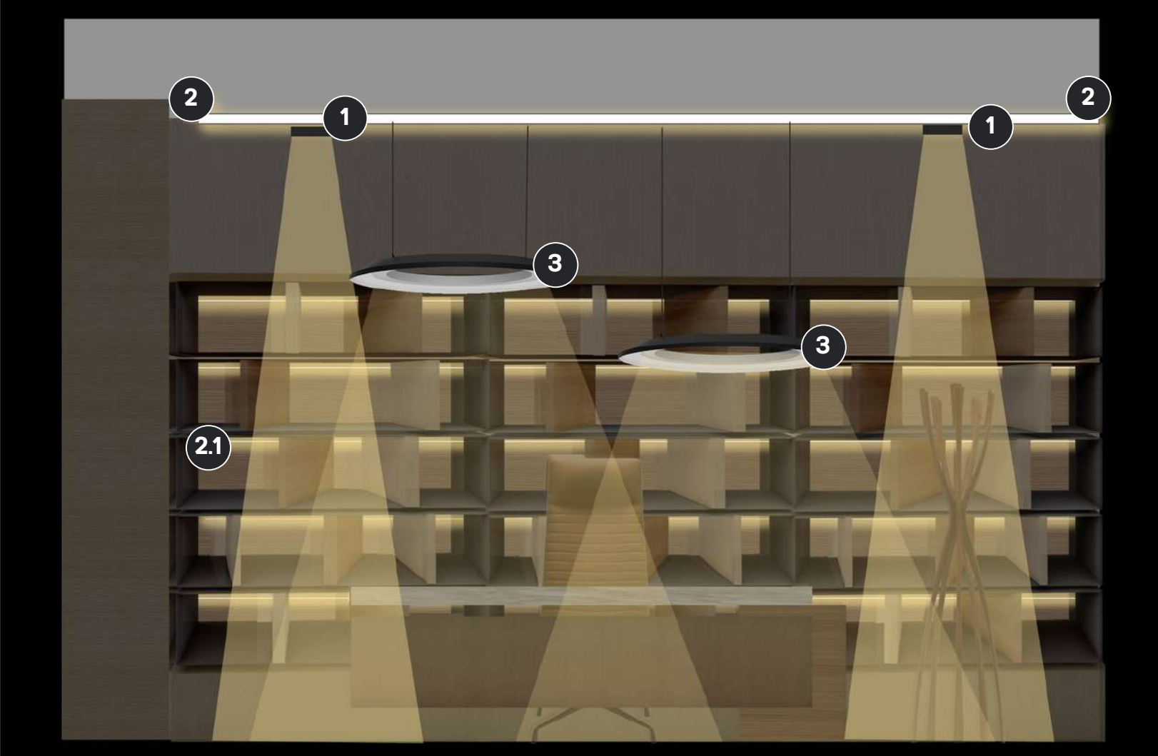
ALZADO 1 ESTUDIO
