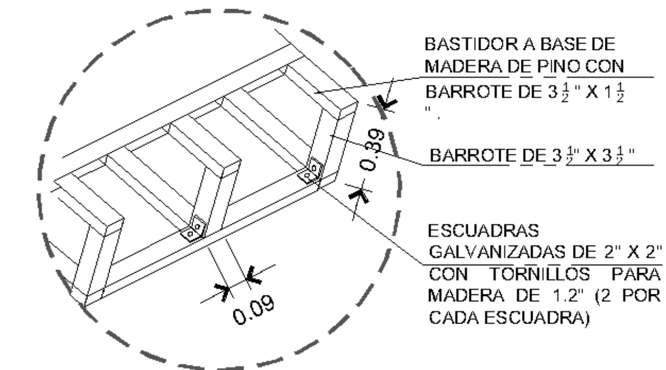
DETALLE A
