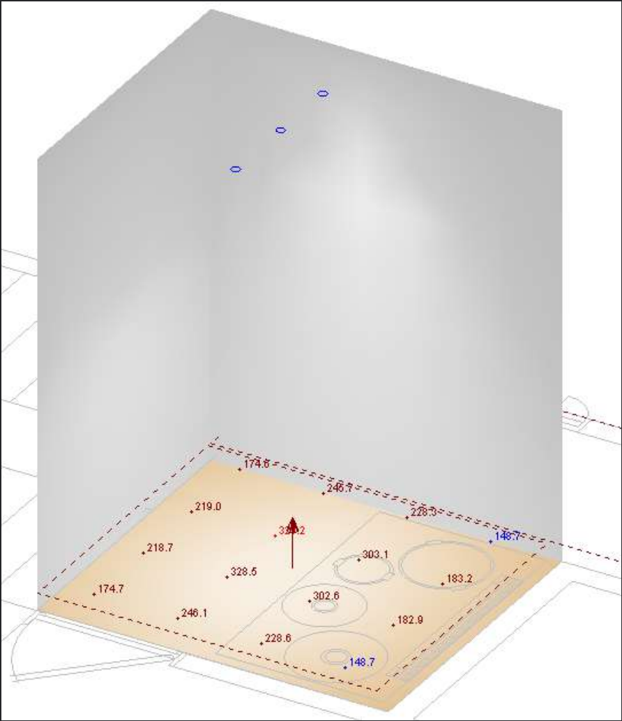
VISTA EN PERSPECTIVA
