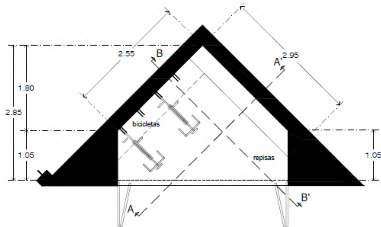
SECCIÓN PLANTA ARQUITECTÓNICA
