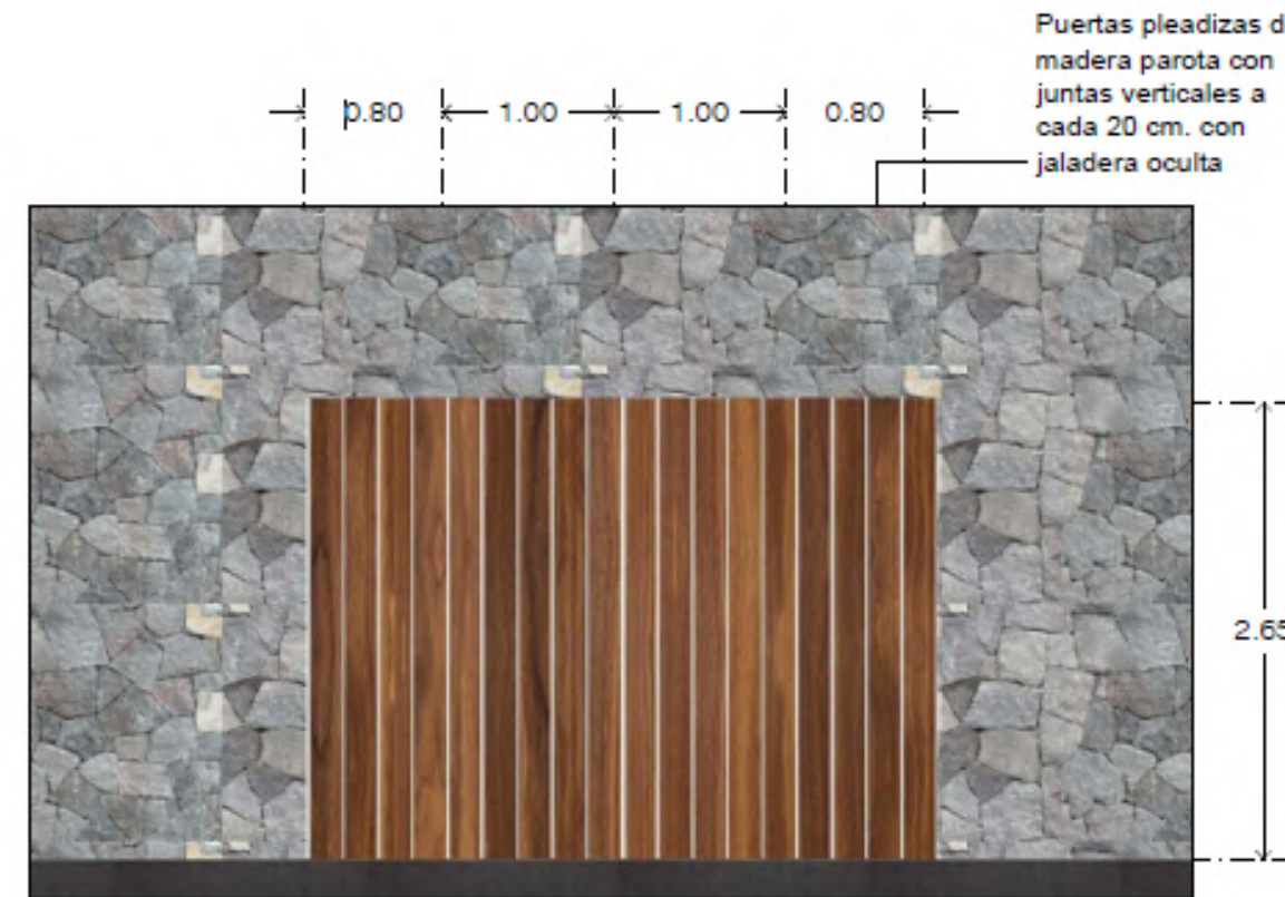
ALZADO FRONTAL EXTERIOR
