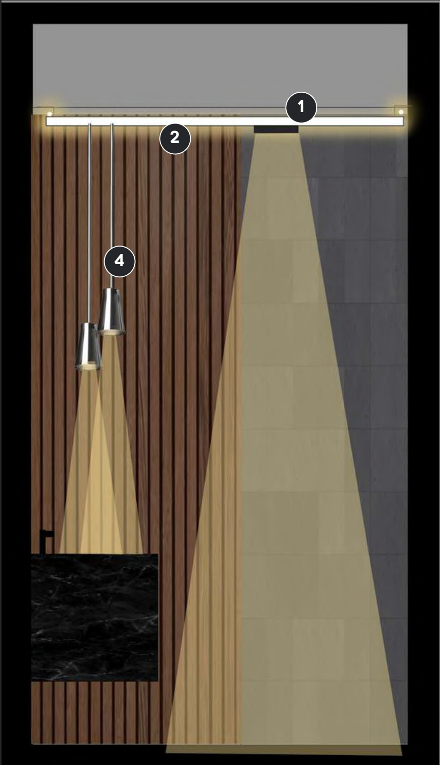
ALZADO 1 BAÑO DE VISITAS
